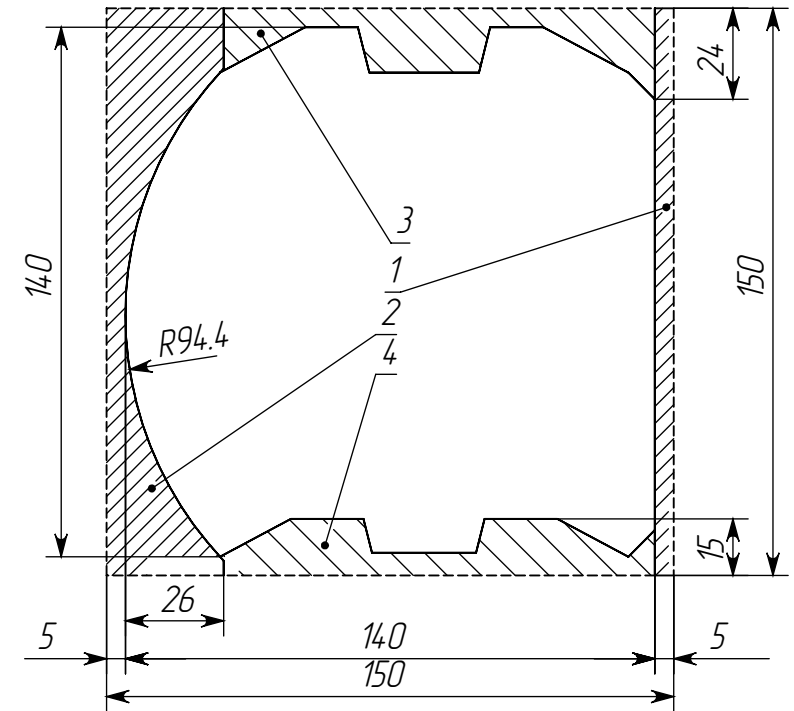
Брус 140x140 мм (заготовка 150x150 мм)
