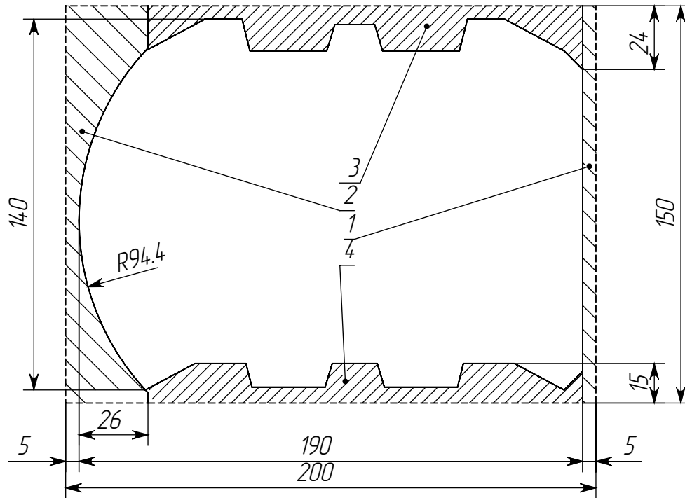
Брус 140x190 мм (заготовка 150x200 мм)
