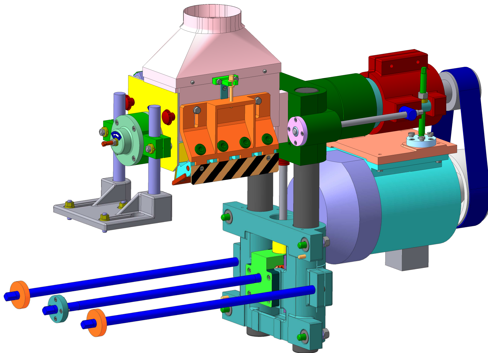
Суппорт верхний С25-4А.15.1.000-01 СБ (лист 1/13)
